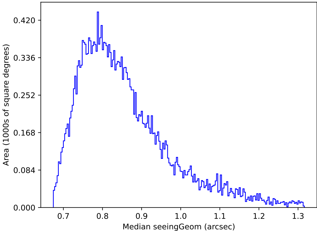
weather_cloudso20v3.4_10yrs Yr 1 r band: Median seeingGeom
