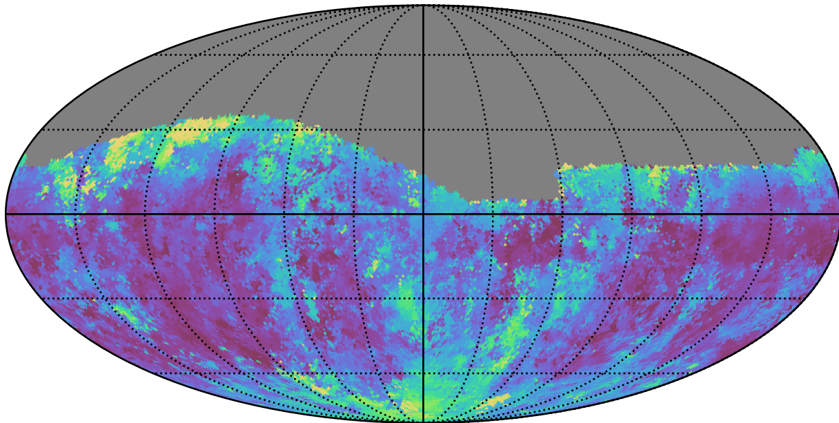
weather_cloudso20v3.4_10yrs Yr 1 g band: Median seeingGeom
