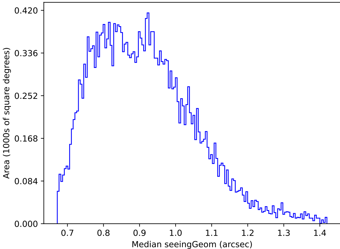
weather_cloudso20v3.4_10yrs Yr 1 g band: Median seeingGeom
