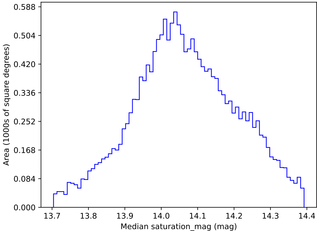
weather_cloudso20v3.4_10yrs WFD z band: Median saturation_mag
