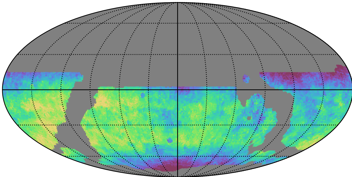
weather_cloudso20v3.4_10yrs WFD y band: Median saturation_mag
