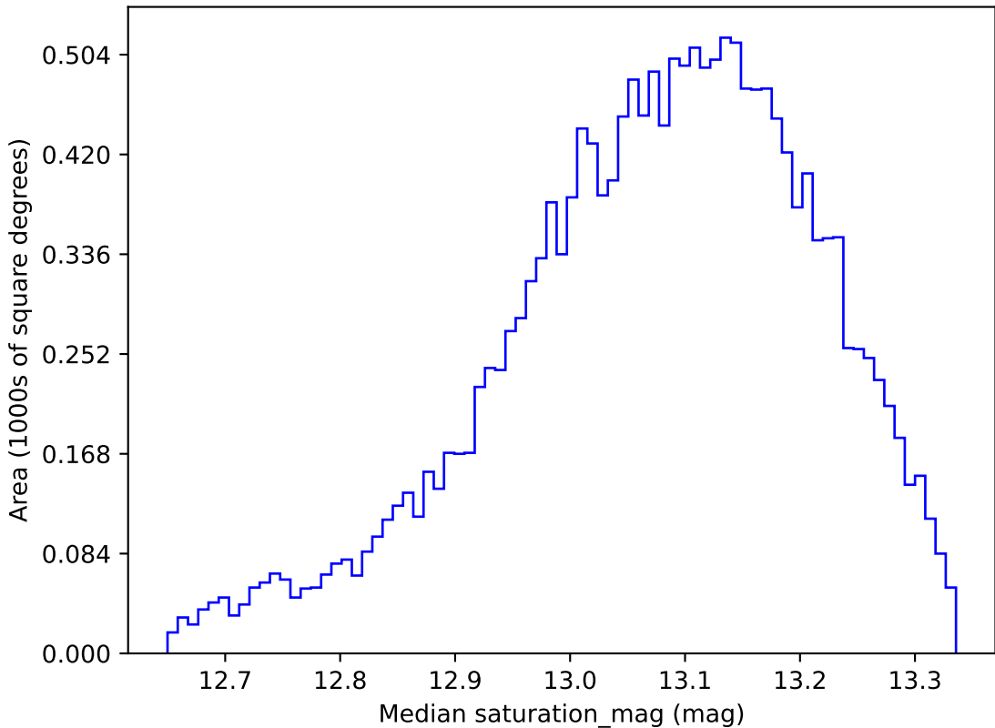
weather_cloudso20v3.4_10yrs WFD y band: Median saturation_mag
