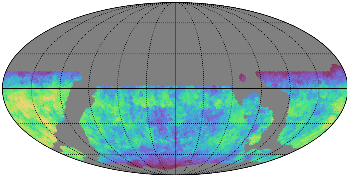
weather_cloudso20v3.4_10yrs WFD u band: Median saturation_mag
