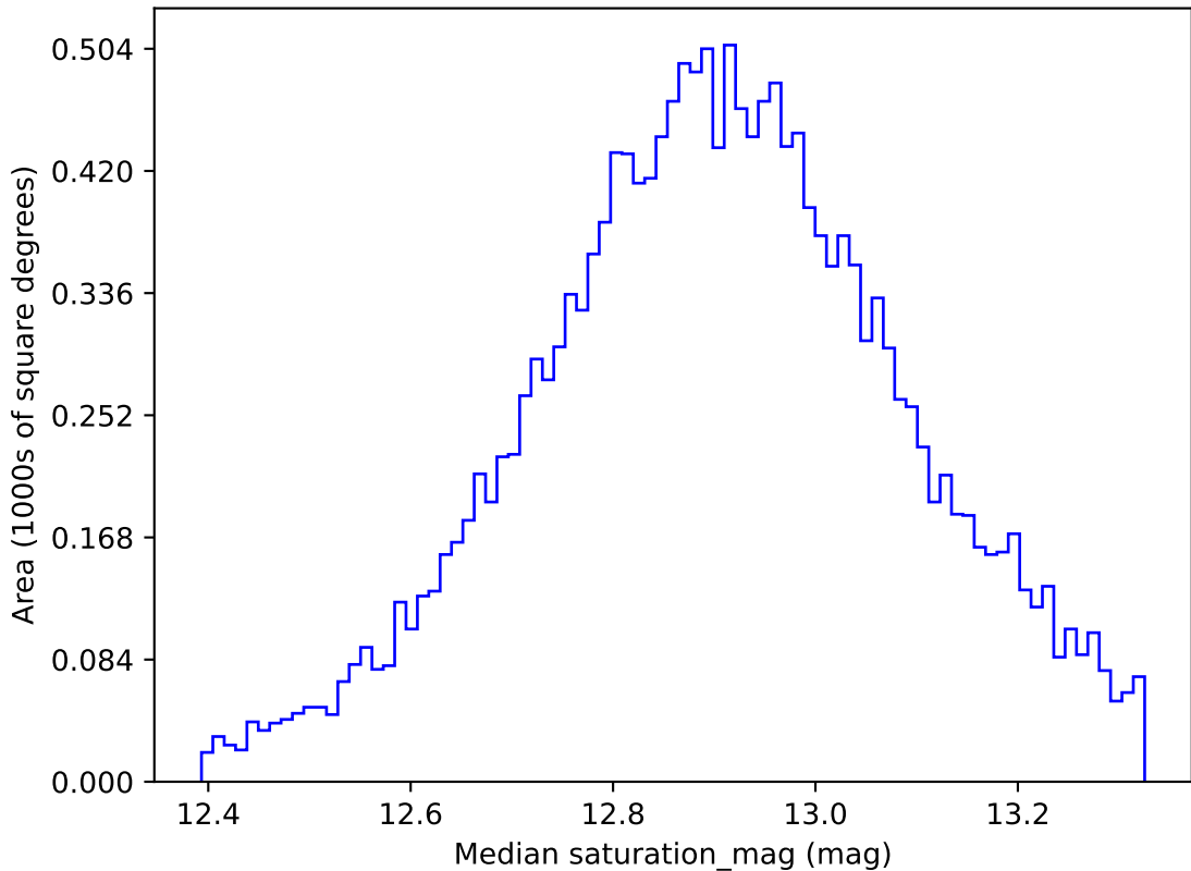
weather_cloudso20v3.4_10yrs WFD u band: Median saturation_mag
