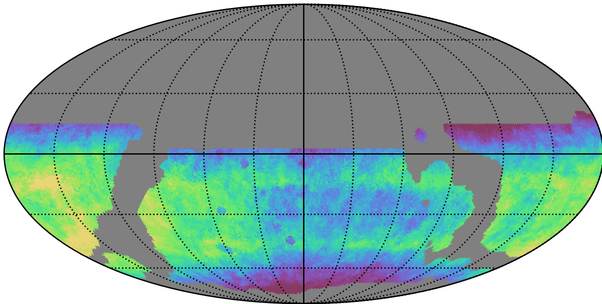
weather_cloudso20v3.4_10yrs WFD r band: Median saturation_mag
