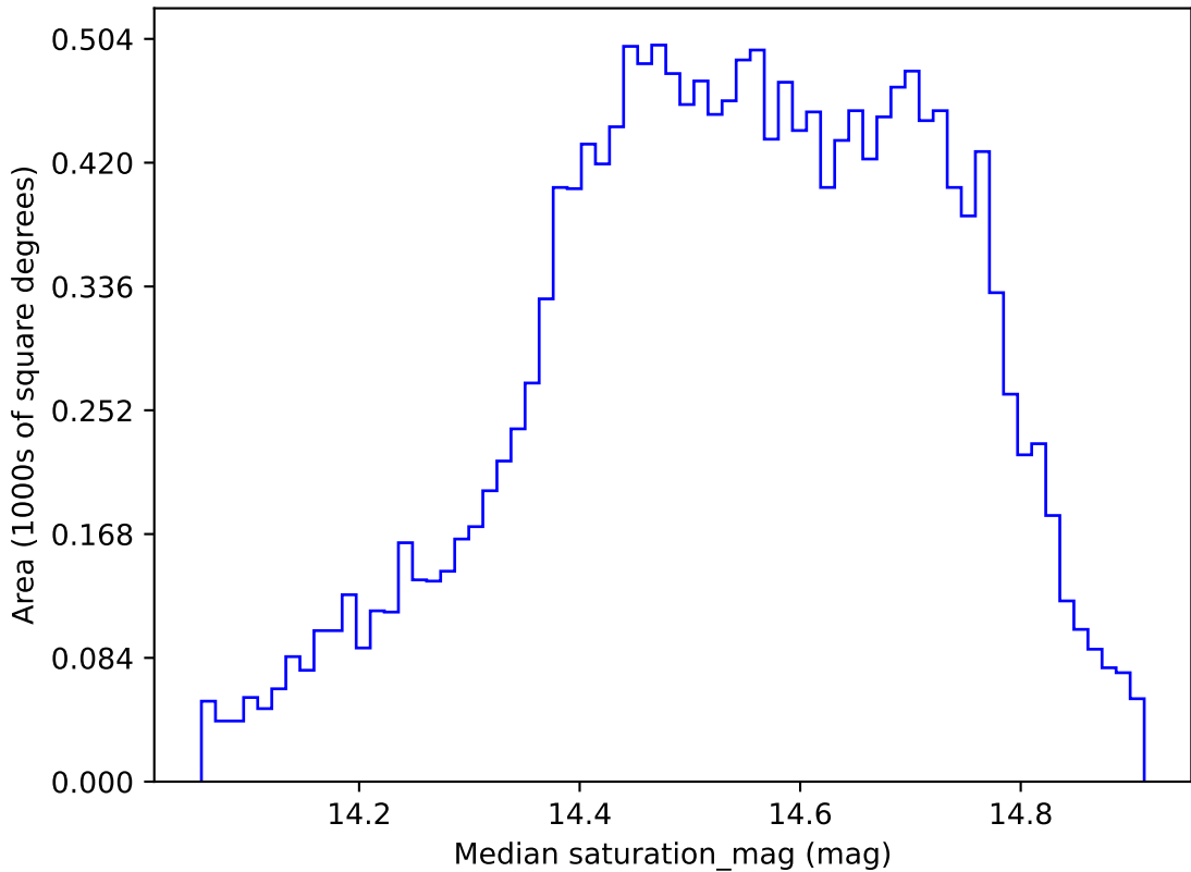
weather_cloudso20v3.4_10yrs WFD r band: Median saturation_mag
