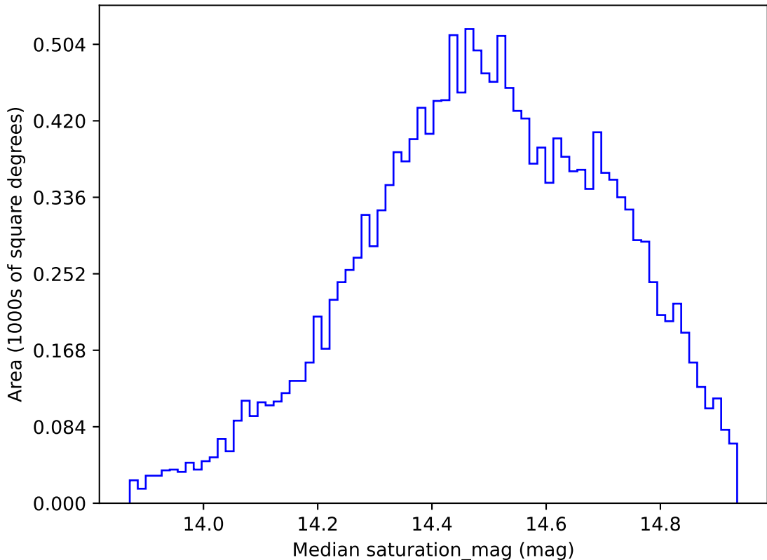
weather_cloudso20v3.4_10yrs WFD g band: Median saturation_mag
