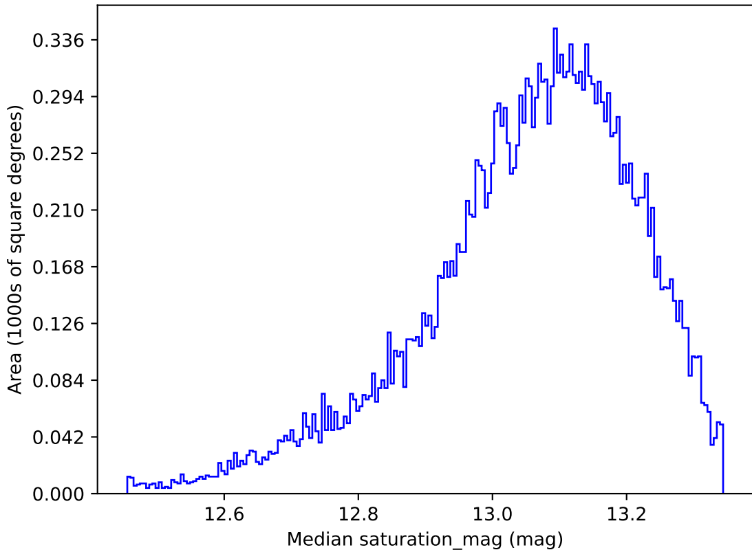
weather_cloudso20v3.4_10yrs All sky y band: Median saturation_mag
