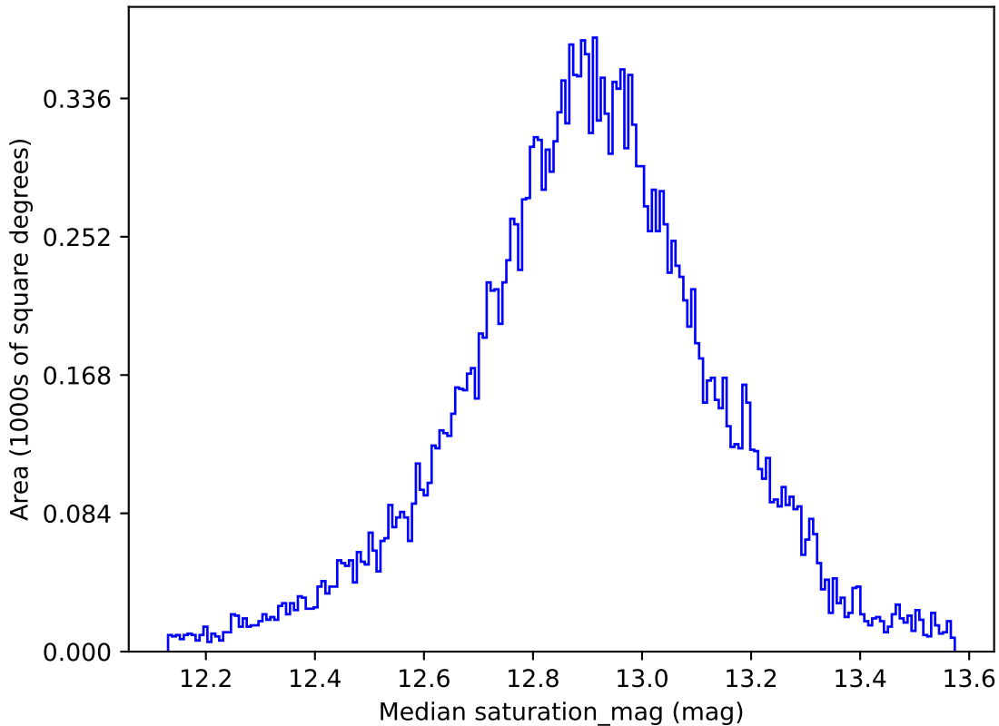
weather_cloudso20v3.4_10yrs All sky u band: Median saturation_mag
