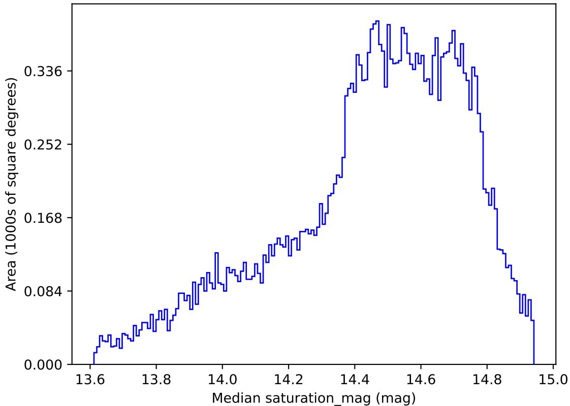
weather_cloudso20v3.4_10yrs All sky r band: Median saturation_mag
