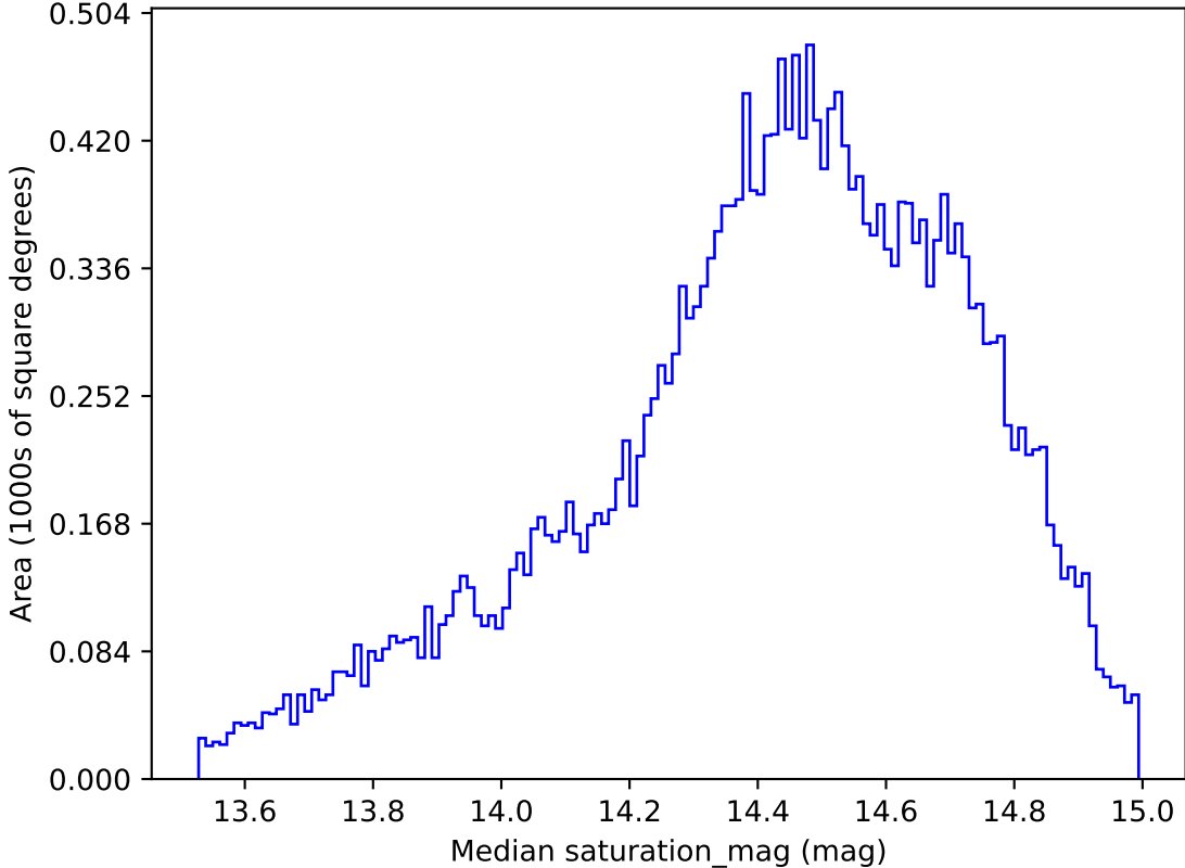
weather_cloudso20v3.4_10yrs All sky g band: Median saturation_mag
