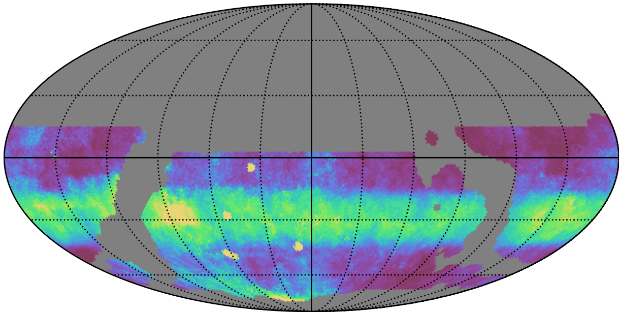
weather_cloudso20v3.4_10yrs WFD z band: Median normairmass
