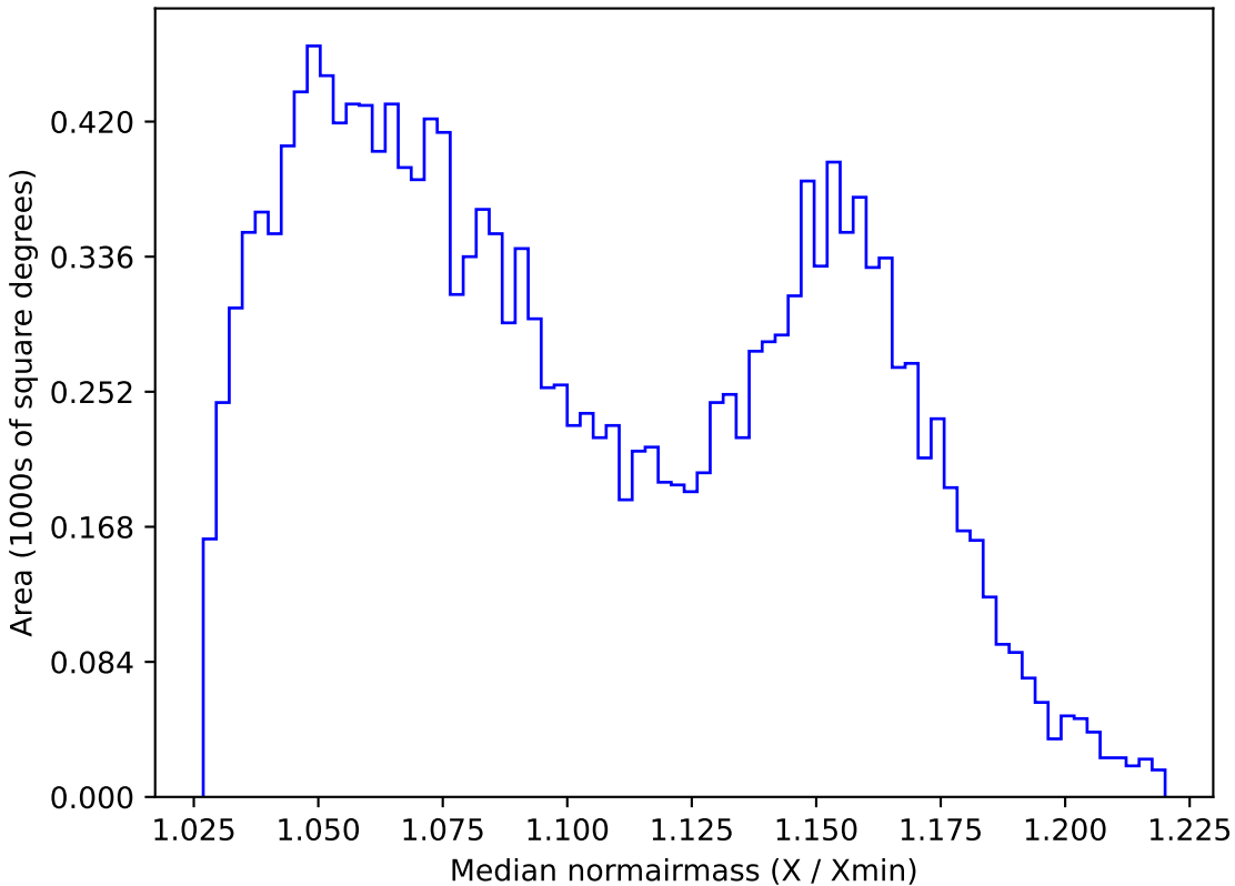
weather_cloudso20v3.4_10yrs WFD z band: Median normairmass
