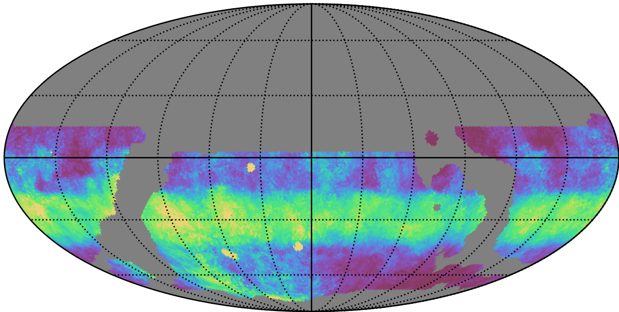
weather_cloudso20v3.4_10yrs WFD y band: Median normairmass
