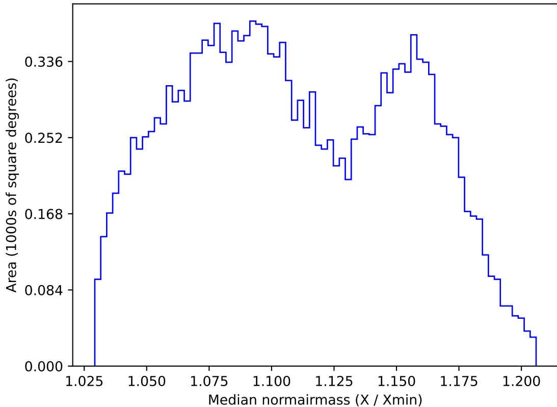
weather_cloudso20v3.4_10yrs WFD y band: Median normairmass
