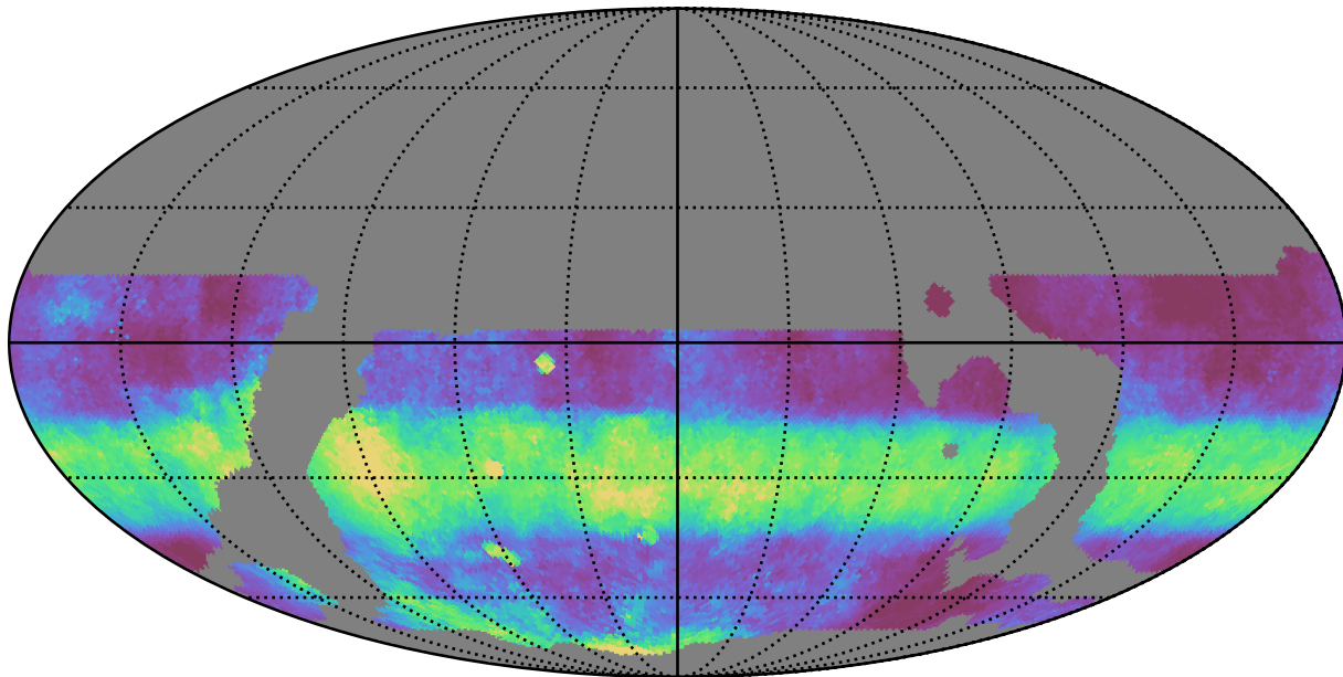
weather_cloudso20v3.4_10yrs WFD i band: Median normairmass
