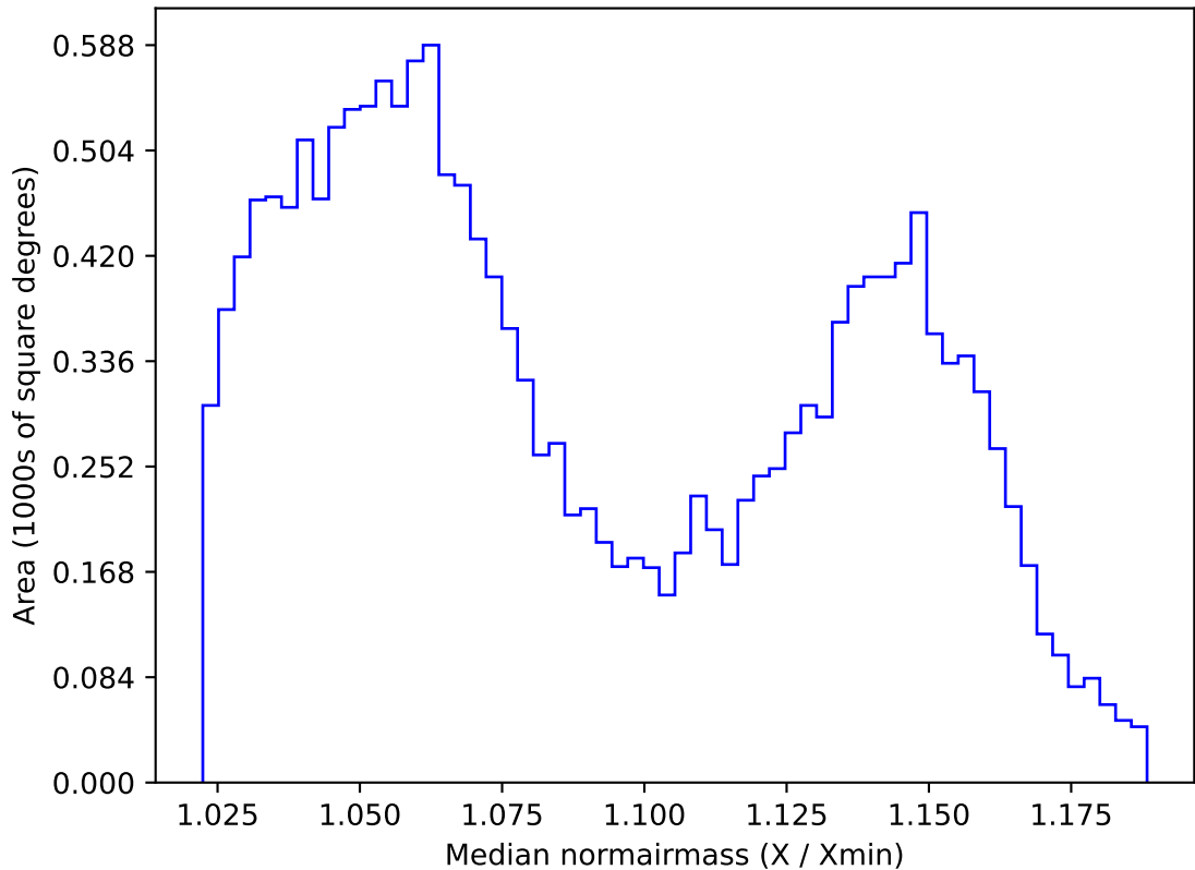
weather_cloudso20v3.4_10yrs WFD i band: Median normairmass
