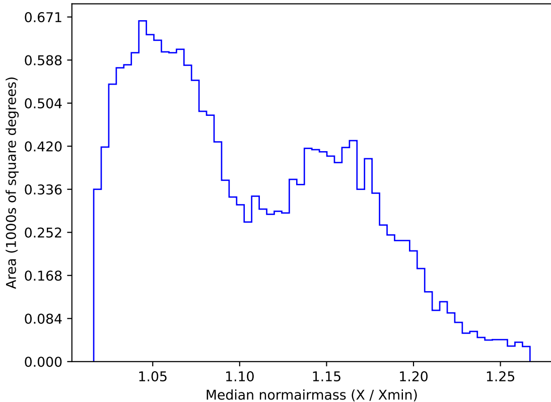
weather_cloudso20v3.4_10yrs WFD g band: Median normairmass
