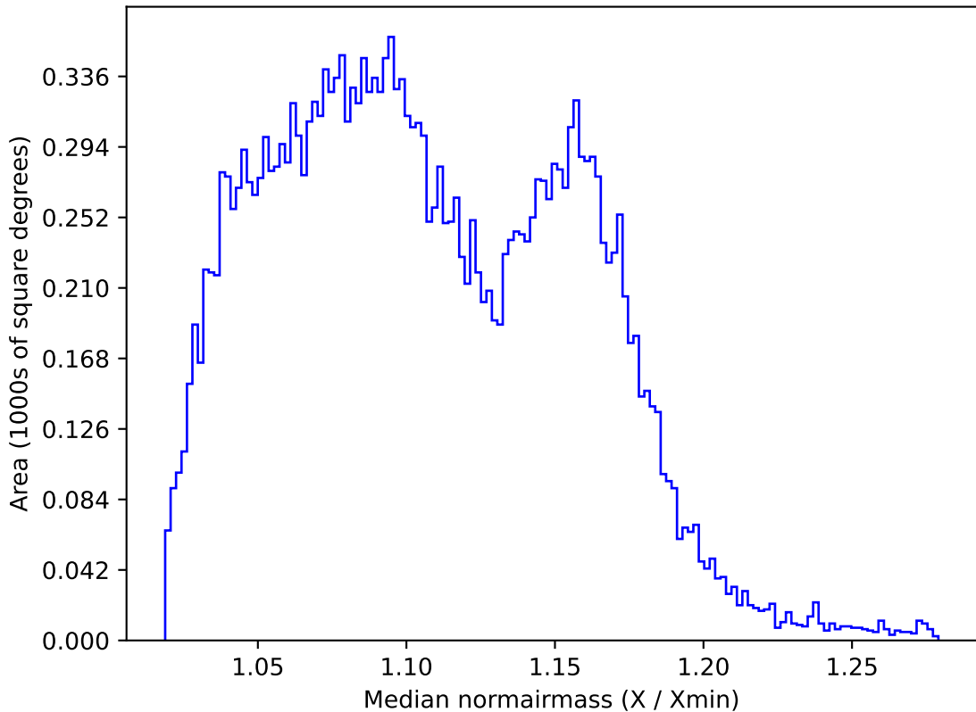
weather_cloudso20v3.4_10yrs All sky y band: Median normairmass
