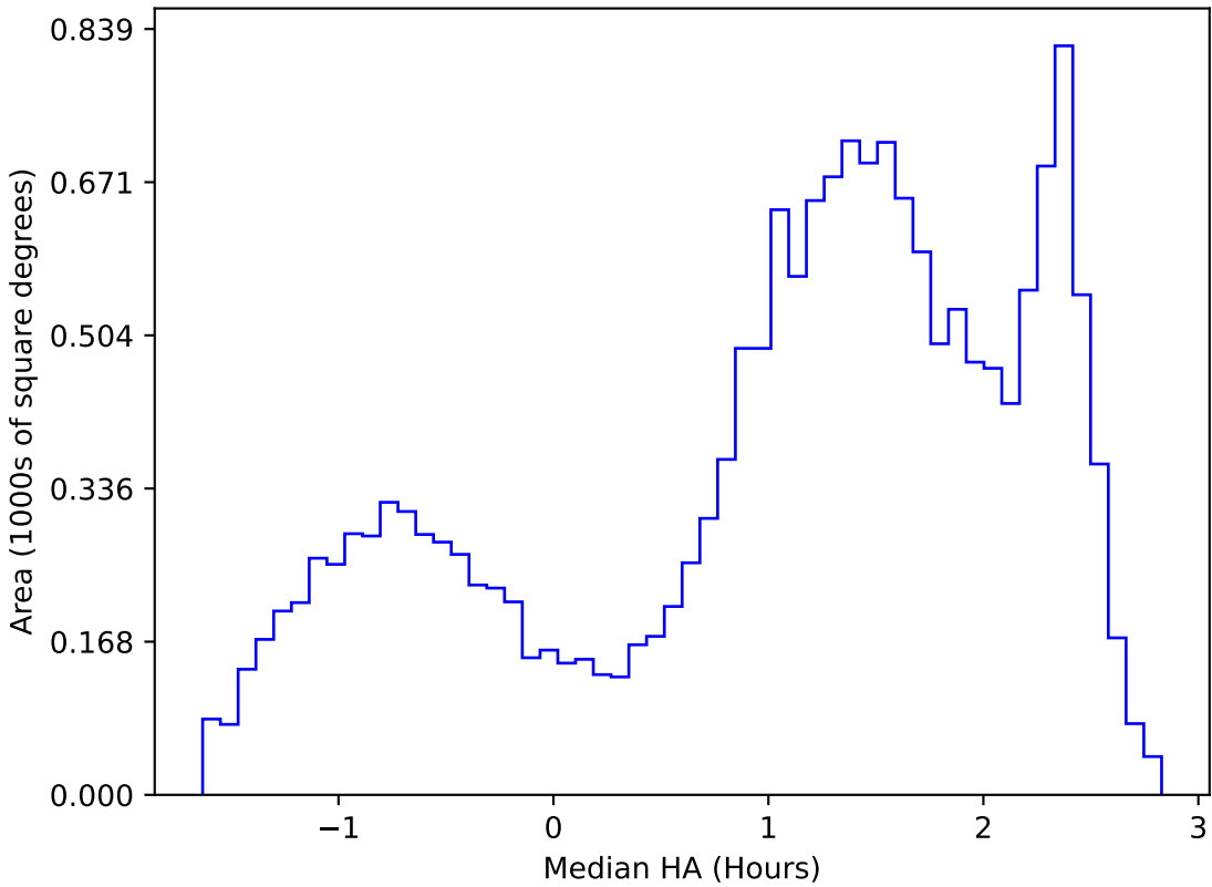
weather_cloudso20v3.4_10yrs WFD y band: Median HA
