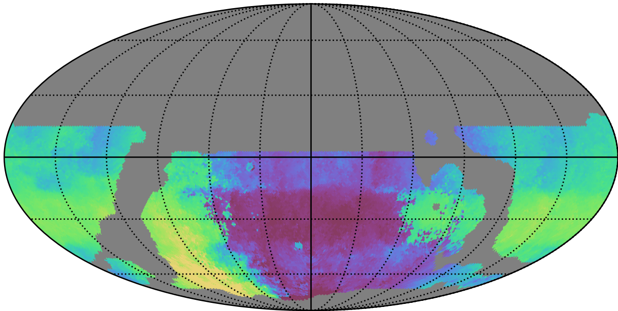
weather_cloudso20v3.4_10yrs WFD u band: Median HA
