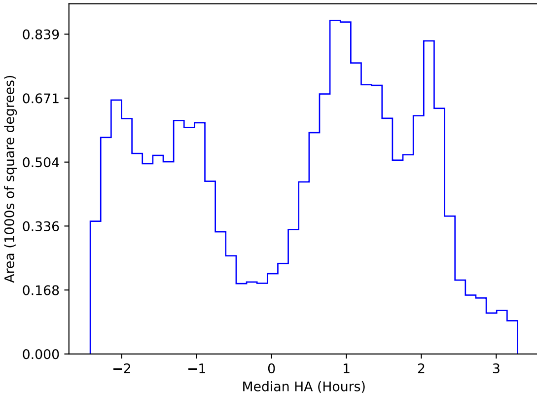
weather_cloudso20v3.4_10yrs WFD u band: Median HA
