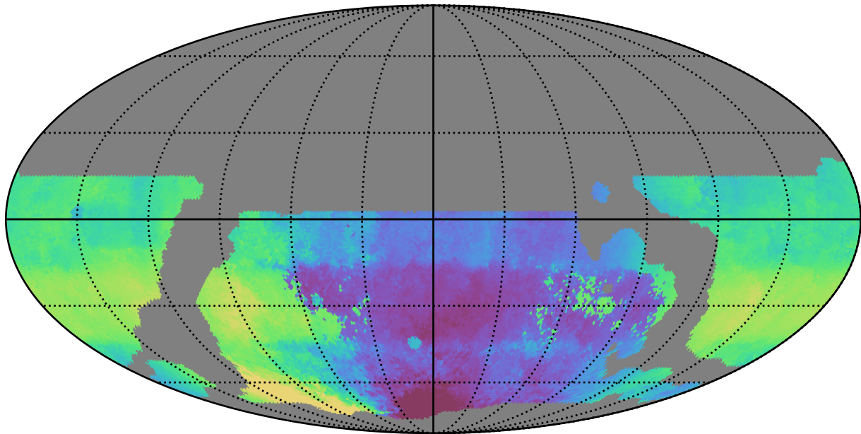
weather_cloudso20v3.4_10yrs WFD g band: Median HA
