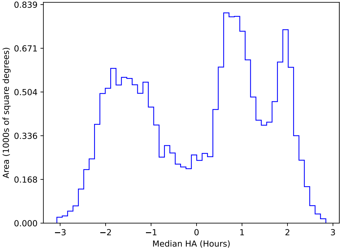
weather_cloudso20v3.4_10yrs WFD g band: Median HA
