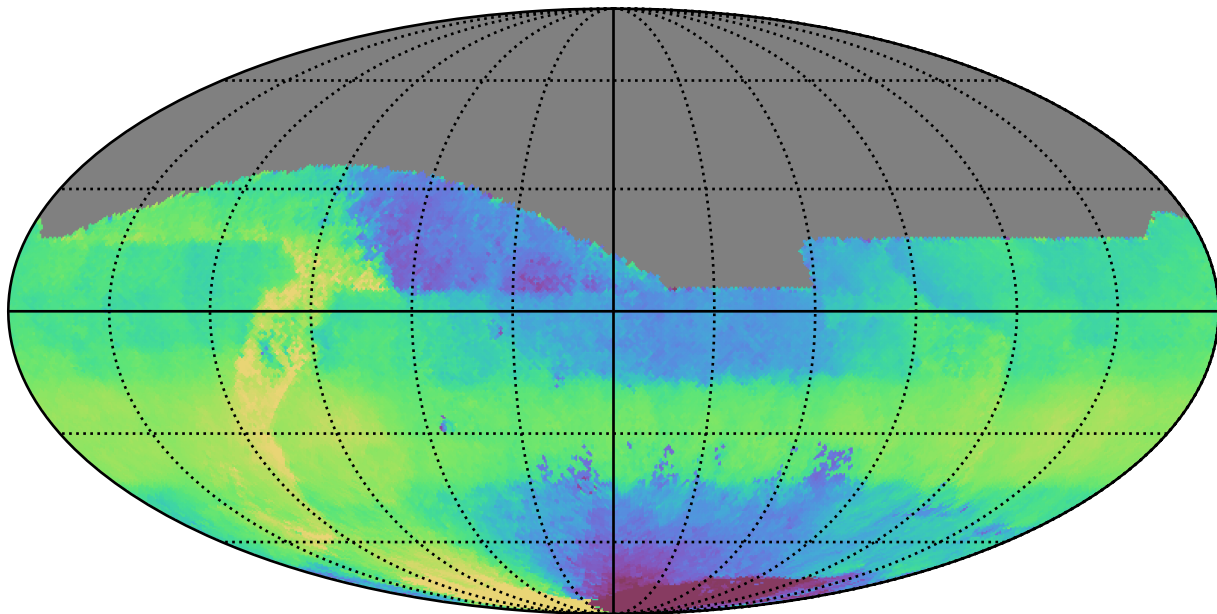
weather_cloudso20v3.4_10yrs All sky z band: Median HA
