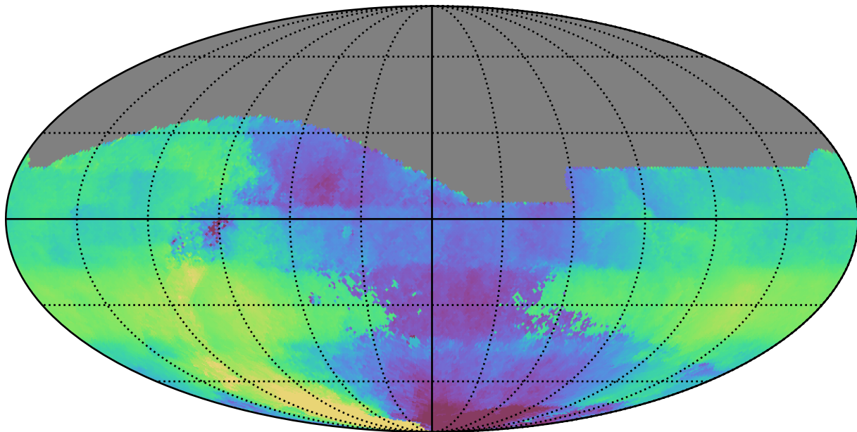
weather_cloudso20v3.4_10yrs All sky r band: Median HA
