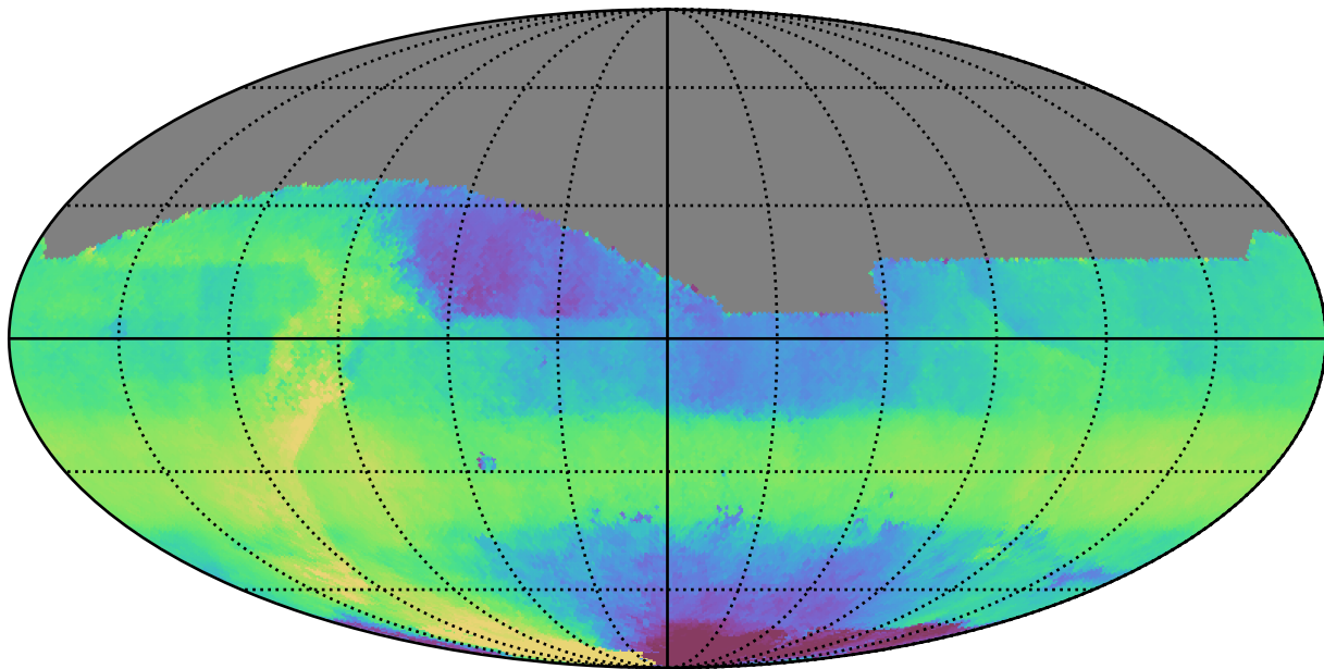
weather_cloudso20v3.4_10yrs All sky i band: Median HA
