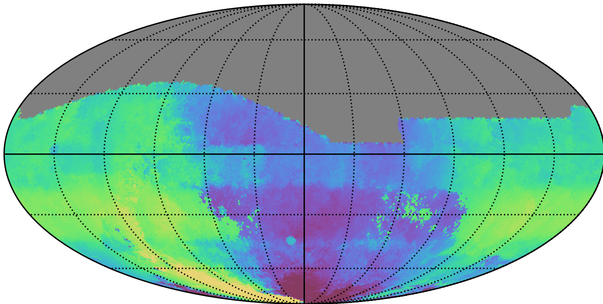
weather_cloudso20v3.4_10yrs All sky g band: Median HA
