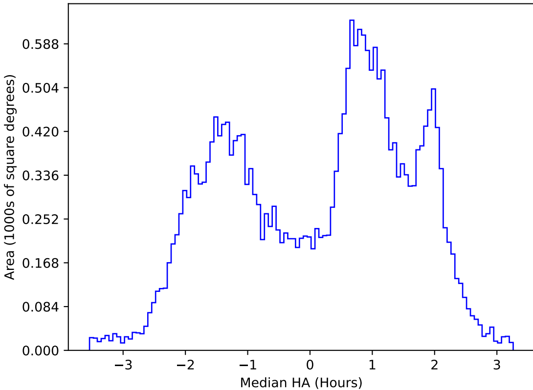
weather_cloudso20v3.4_10yrs All sky g band: Median HA
