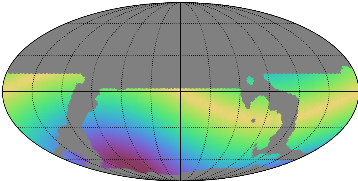
weather_cloudso20v3.4_10yrs WFD z band: Max solarElong
