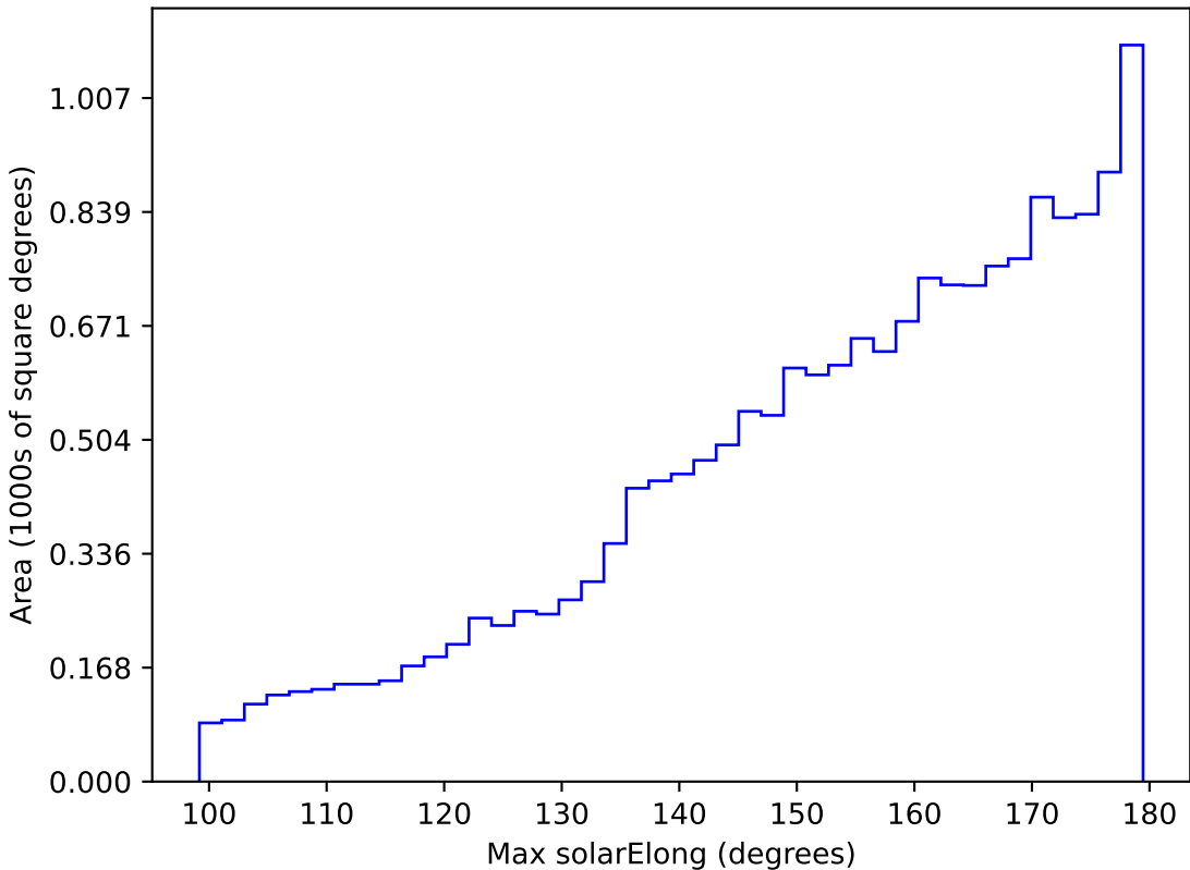
weather_cloudso20v3.4_10yrs WFD z band: Max solarElong
