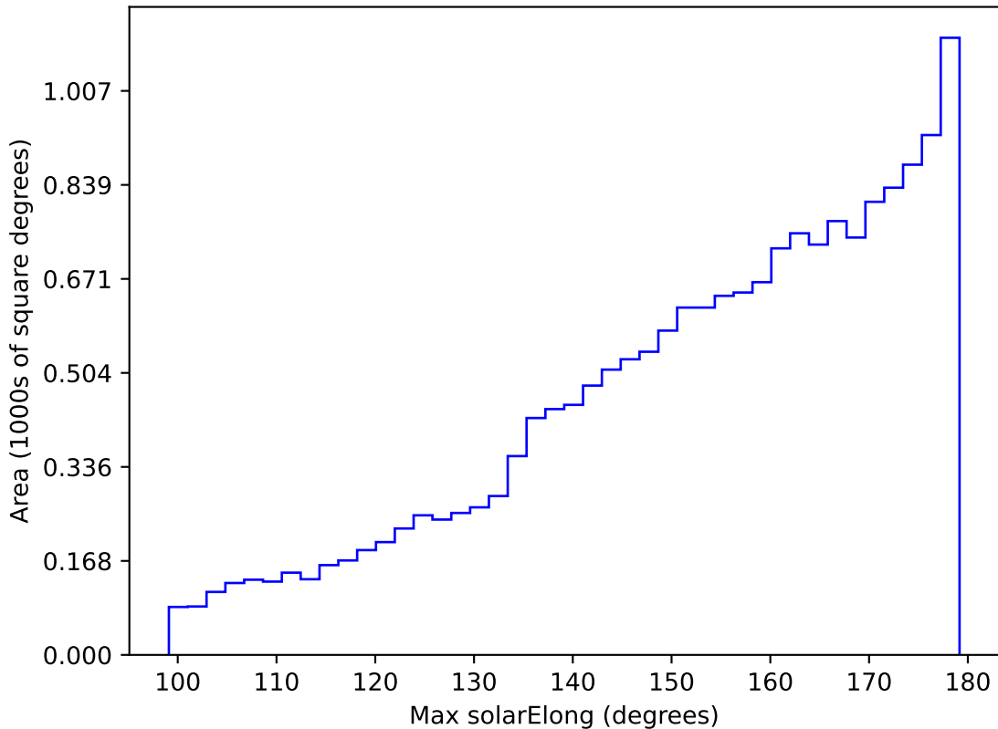
weather_cloudso20v3.4_10yrs WFD y band: Max solarElong
