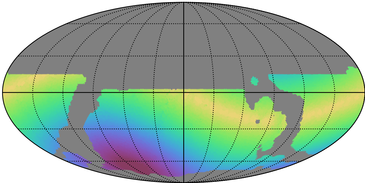
weather_cloudso20v3.4_10yrs WFD u band: Max solarElong
