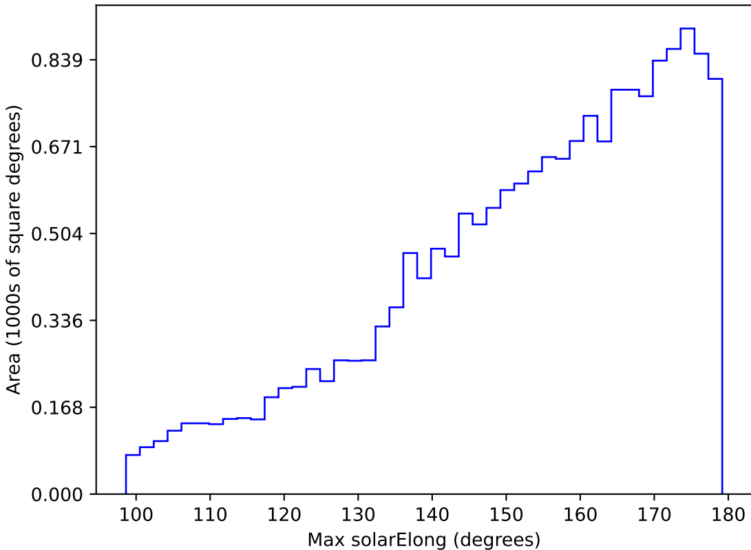
weather_cloudso20v3.4_10yrs WFD u band: Max solarElong
