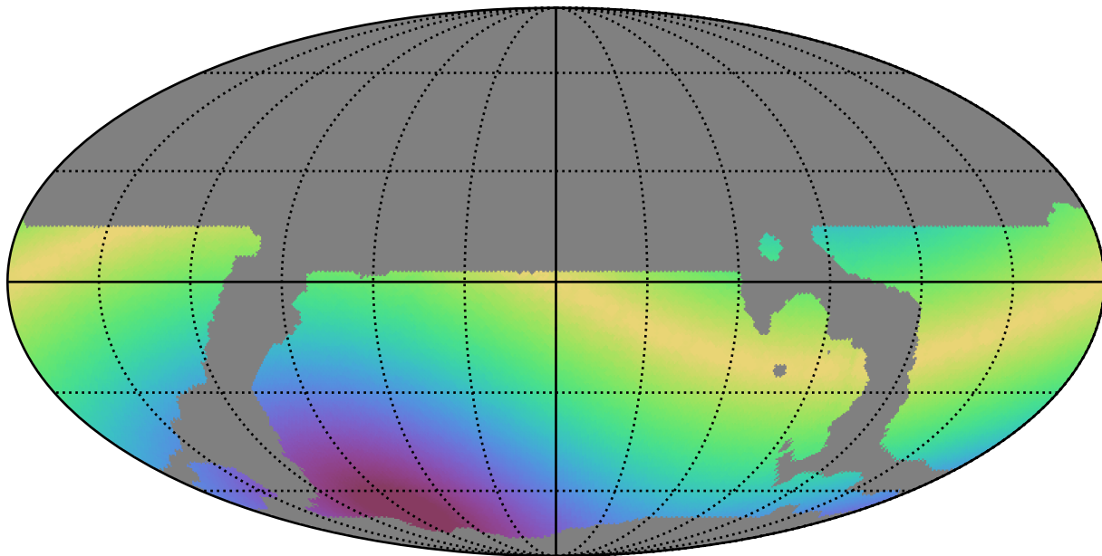
weather_cloudso20v3.4_10yrs WFD r band: Max solarElong
