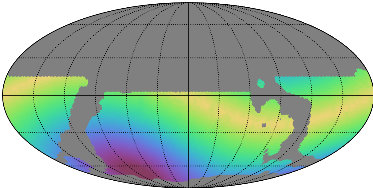
weather_cloudso20v3.4_10yrs WFD g band: Max solarElong
