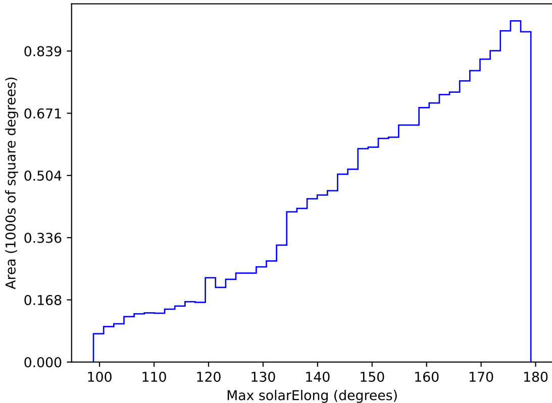
weather_cloudso20v3.4_10yrs WFD g band: Max solarElong
