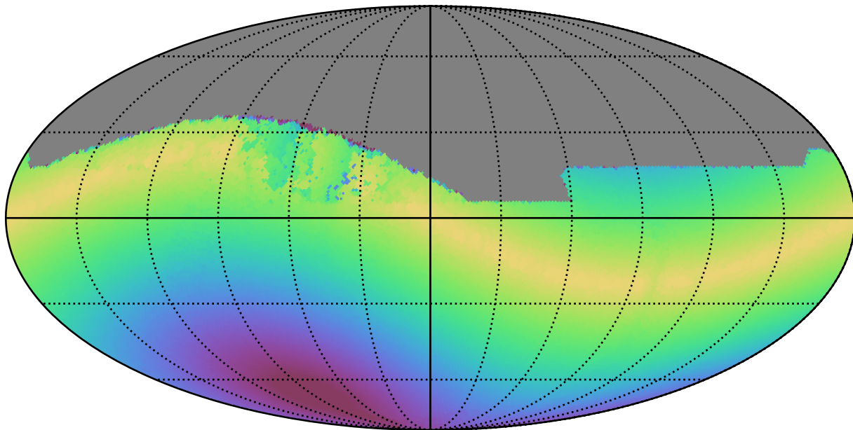
weather_cloudso20v3.4_10yrs All sky z band: Max solarElong
