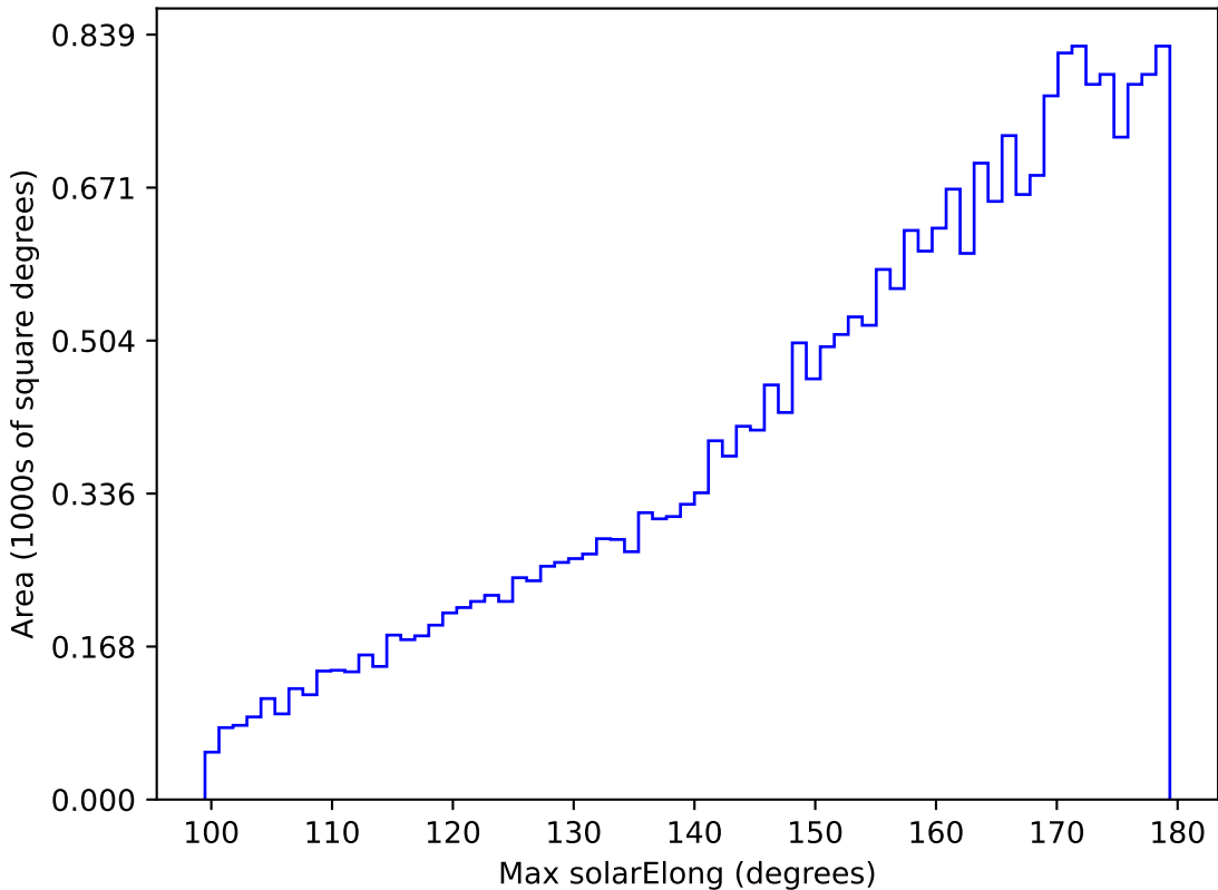
weather_cloudso20v3.4_10yrs All sky z band: Max solarElong
