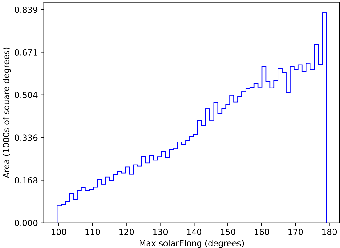
weather_cloudso20v3.4_10yrs All sky y band: Max solarElong
