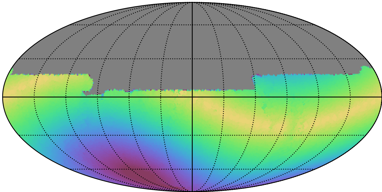
weather_cloudso20v3.4_10yrs All sky u band: Max solarElong
