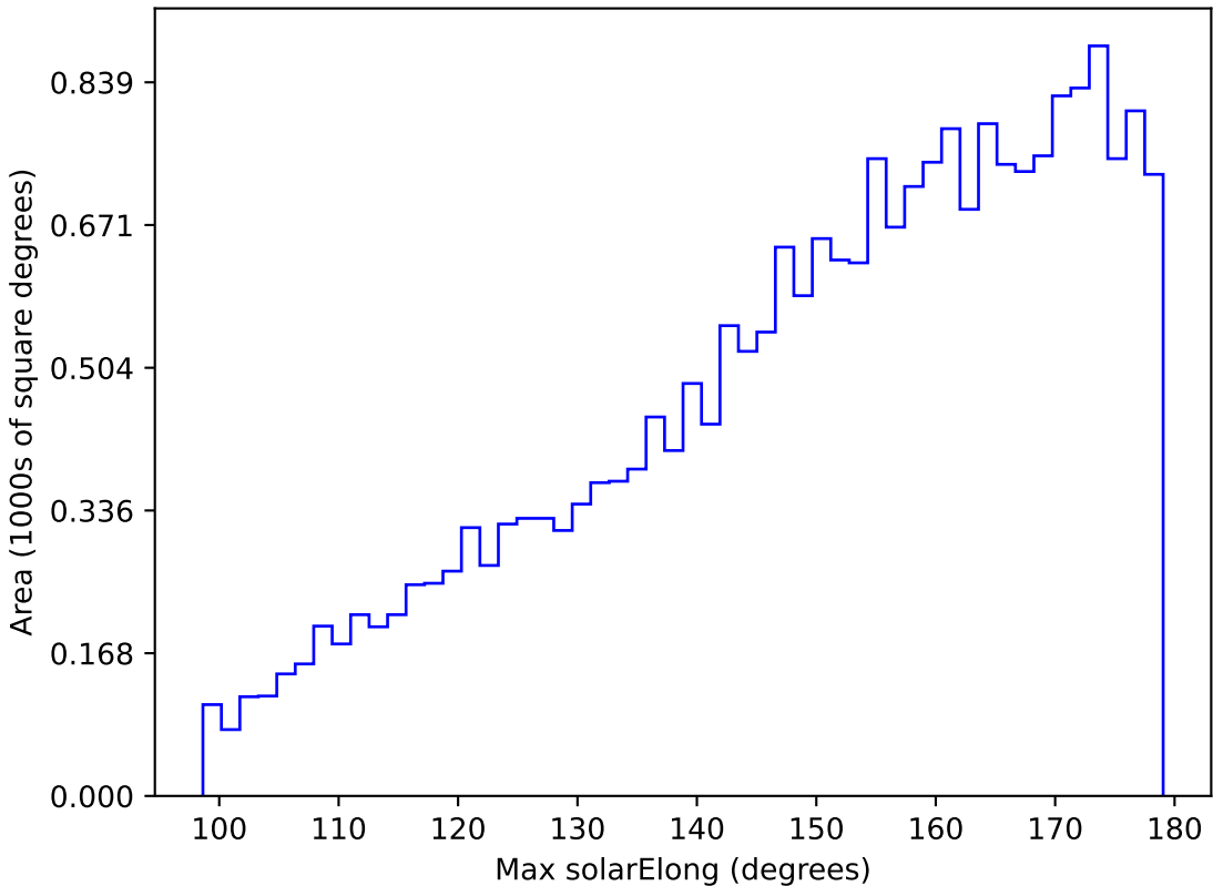
weather_cloudso20v3.4_10yrs All sky u band: Max solarElong
