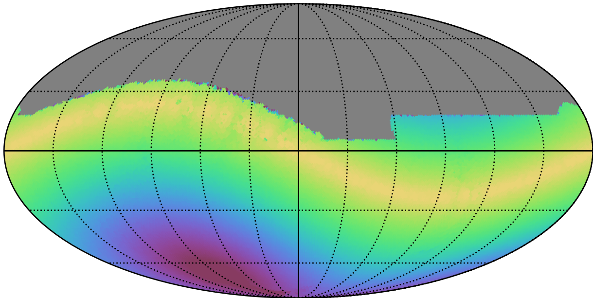
weather_cloudso20v3.4_10yrs All sky r band: Max solarElong
