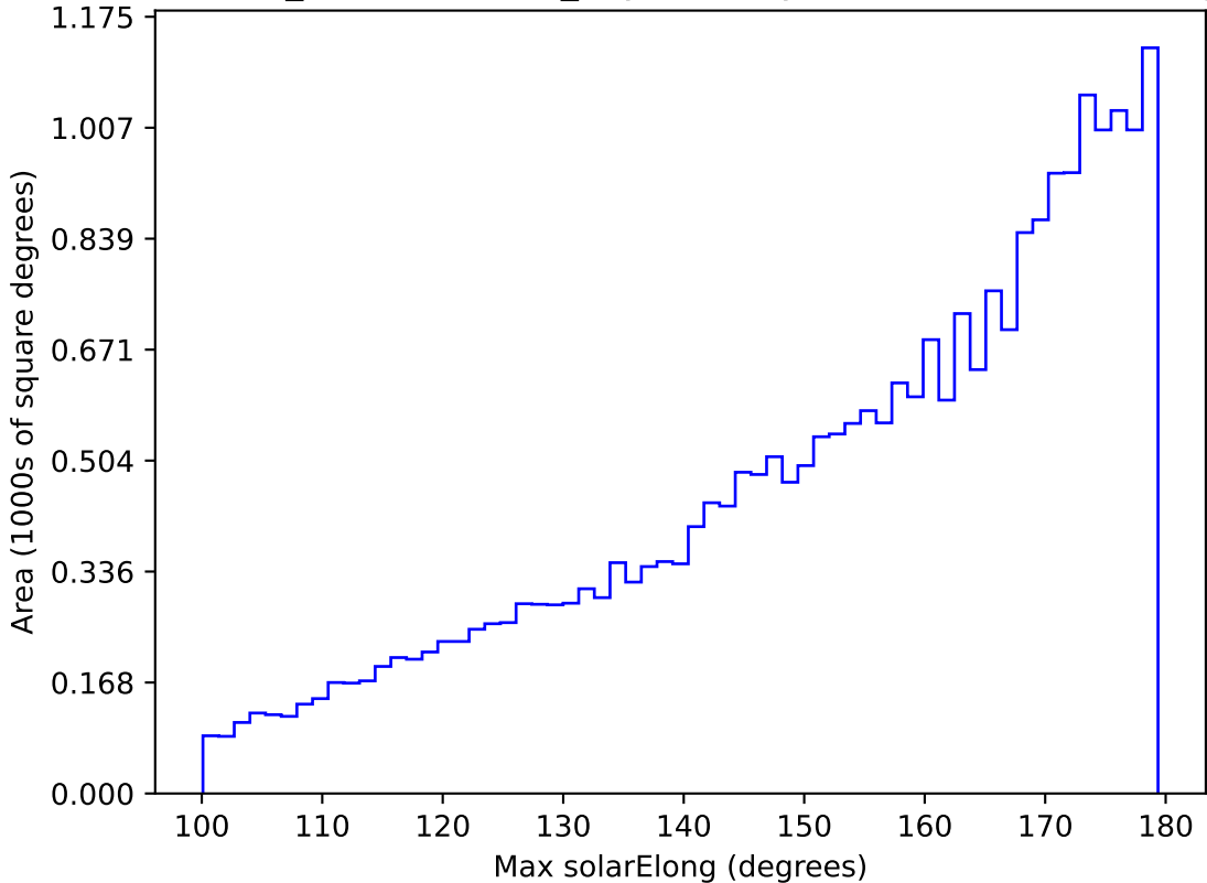
weather_cloudso20v3.4_10yrs All sky r band: Max solarElong
