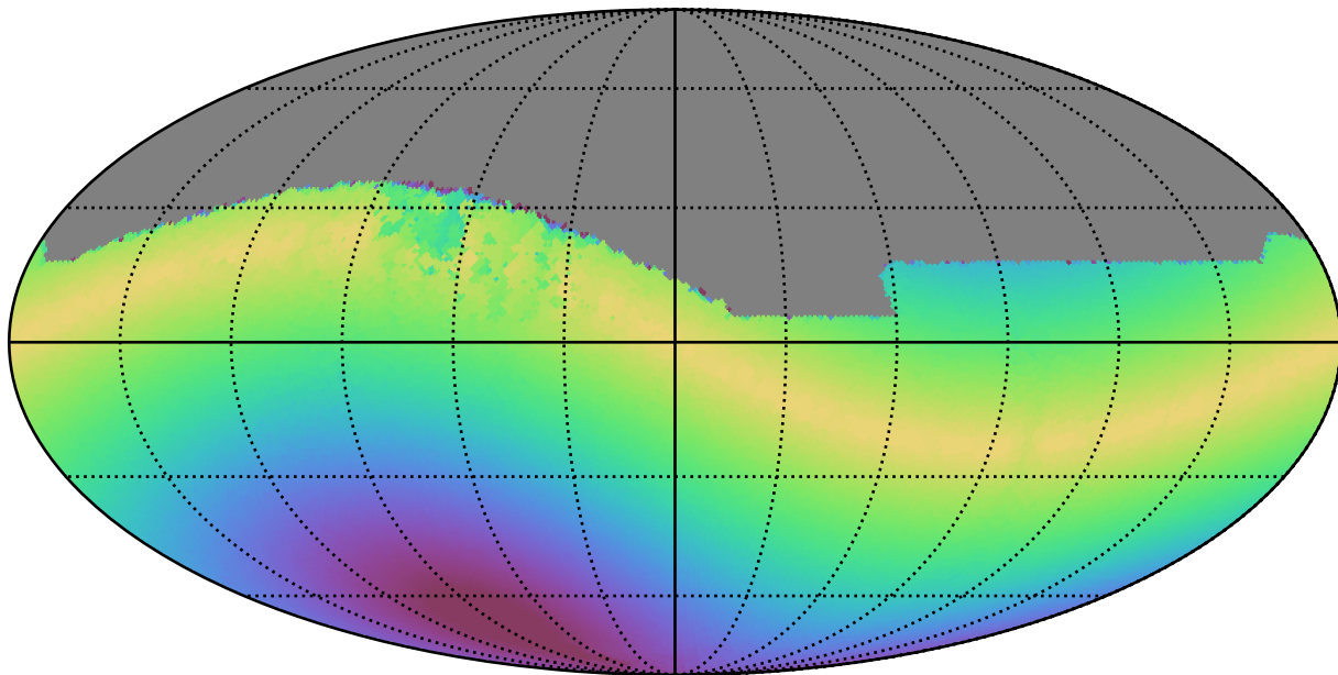
weather_cloudso20v3.4_10yrs All sky i band: Max solarElong
