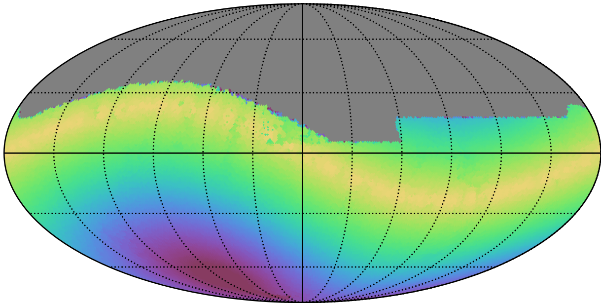
weather_cloudso20v3.4_10yrs All sky g band: Max solarElong
